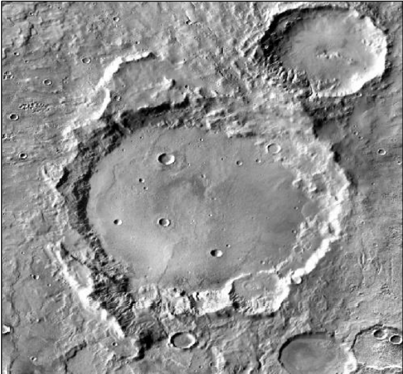
De Cruls krater op Mars. (Foto: Mars Odyssey Orbiter)
